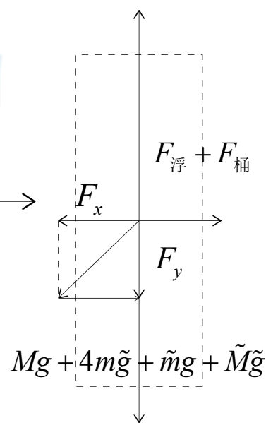
图3 整体法受力分析示意图
