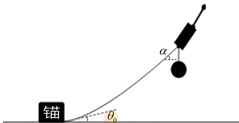
图 6 锚链全部悬空的情形示意图
