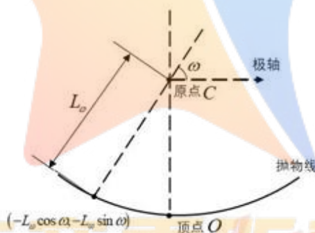
图 2：极坐标系下抛物线示意图
