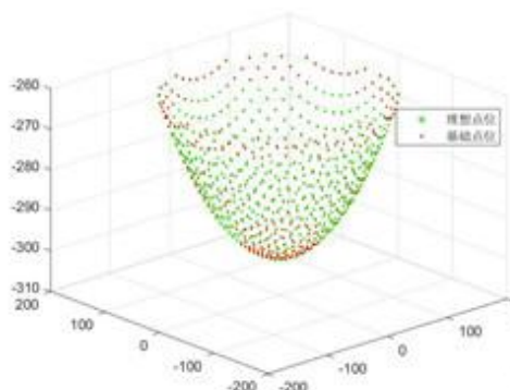
图 13 理想抛物面与基准球面主索节点变化
