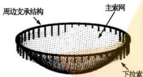
图 1 FAST 主动反射面轴侧图
