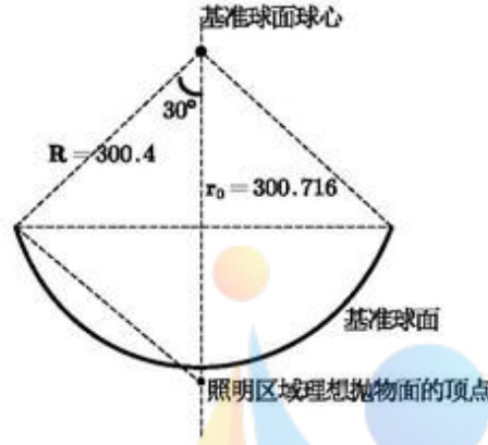
图 16 照明区域基准球面的几何关系
