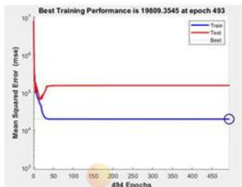
图 5.4-3: 第 493 代时最优训练效果
