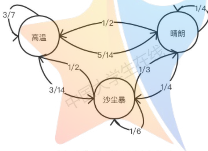
图 8 天气跳转问题的状态转移图
