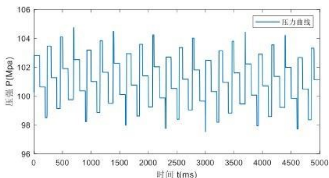
图 19 压强变化图
