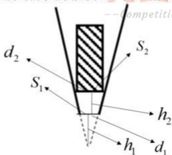
图 16 针阀未上升时
