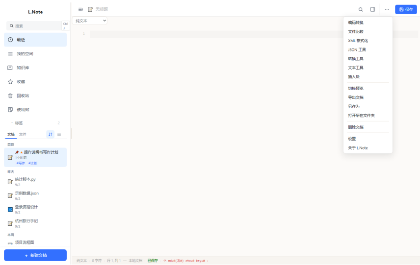
图：导出/另存为入口
