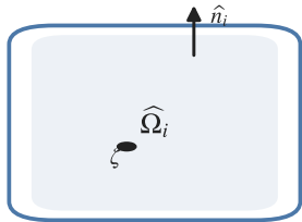
Gradient pullback
