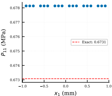
(d) Task 4: incremental loading
