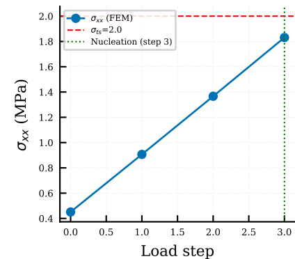
(d) Task 4: incremental loading
