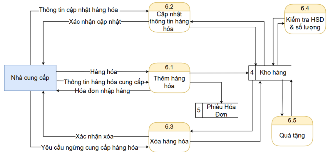
Hình 9: DFD mức 1 – Quản lý hàng hóa
