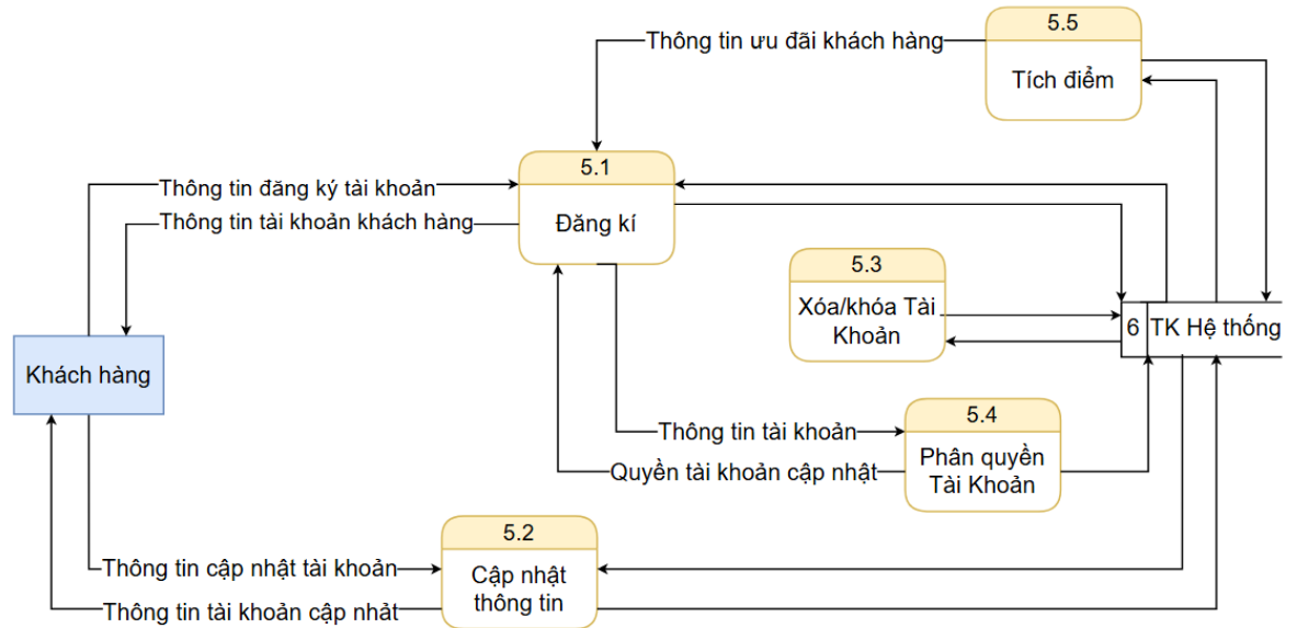
Hình 7: DFD mức 1 – Quản lý tài khoản
