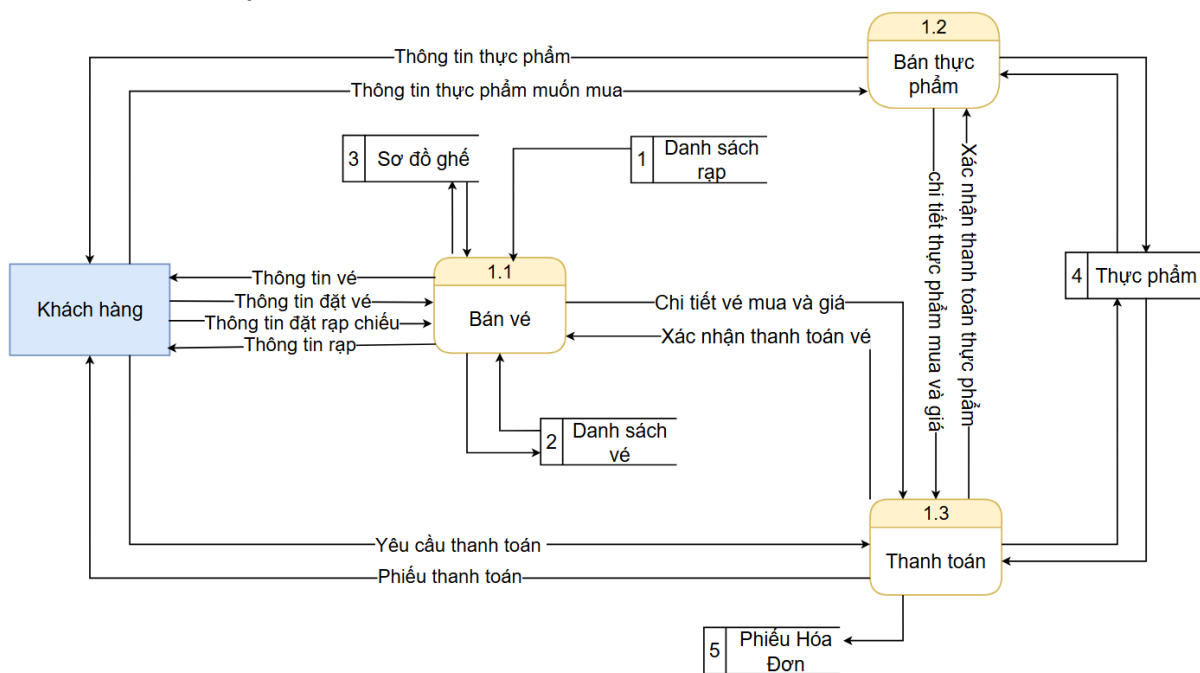
Hình 5: DFD mức 1 – Quản lý dịch vụ
