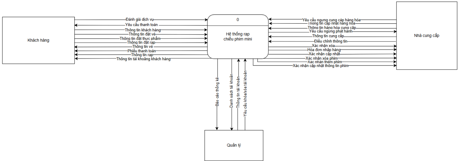
Hình 3: DFD mức ngữ cảnh
