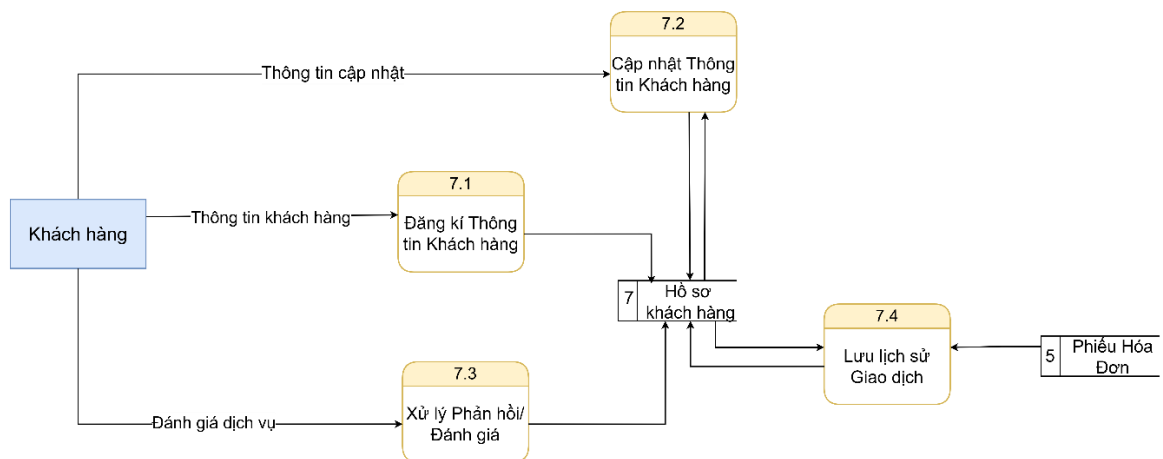
Hình 8: DFD mức 1 – Quản lý khách hàng
