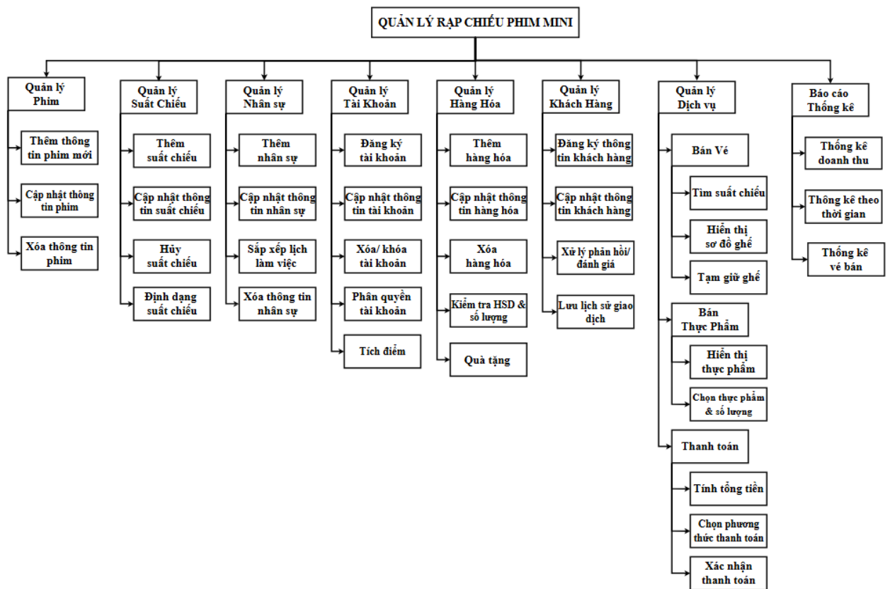
Hình 1: Mô hình phân rã
