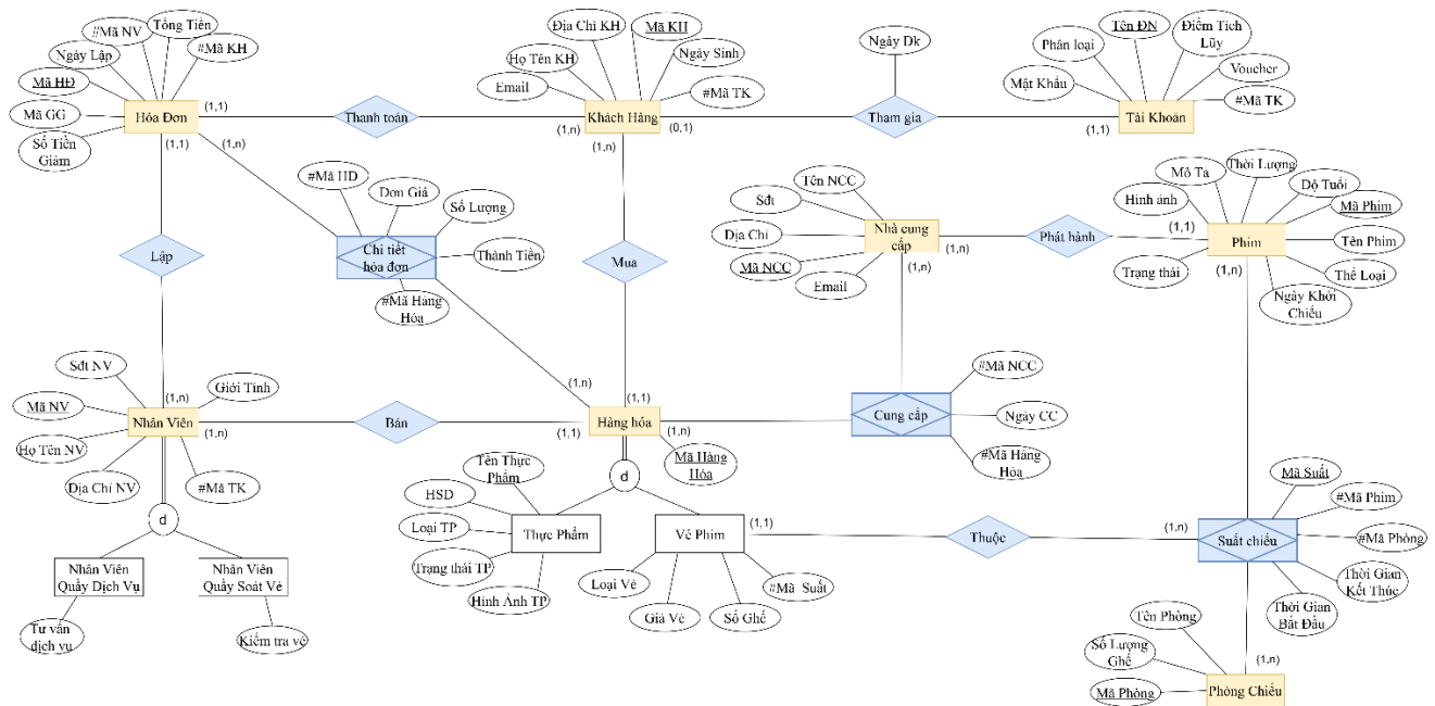
Hình 2: Mô hình ERD
