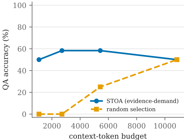
LoCoMo accuracy vs budget (substring (proxy))
