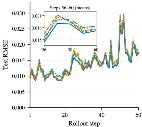
a PFLOTRAN
