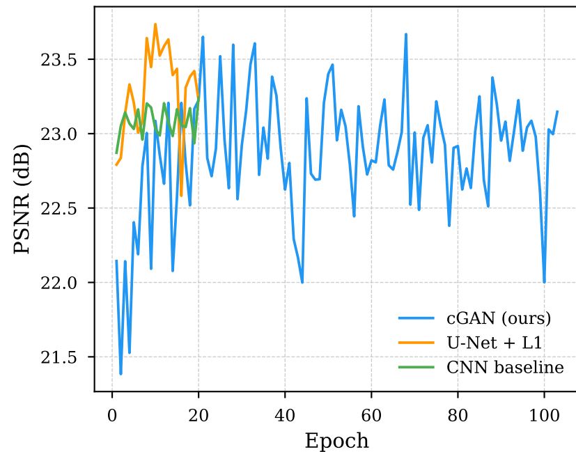
(b) PSNR
