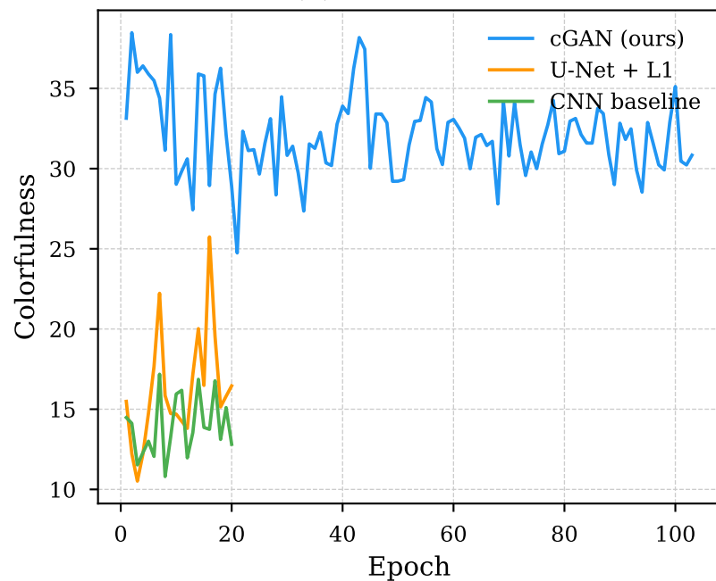
(d) Colorfulness
