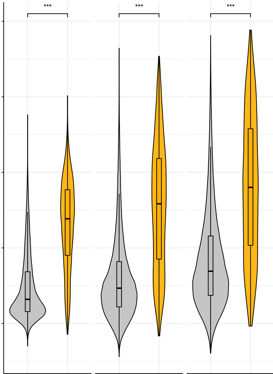
Tajima's D
