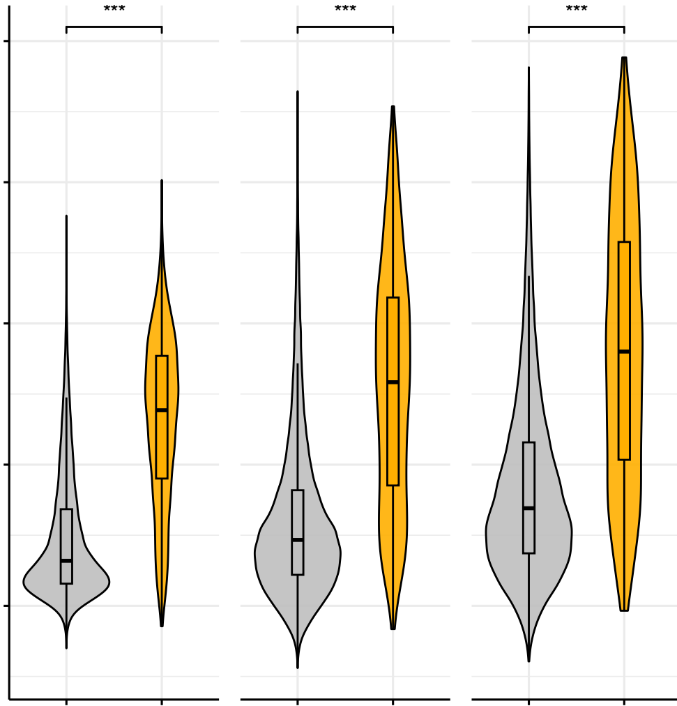
Tajima's D
