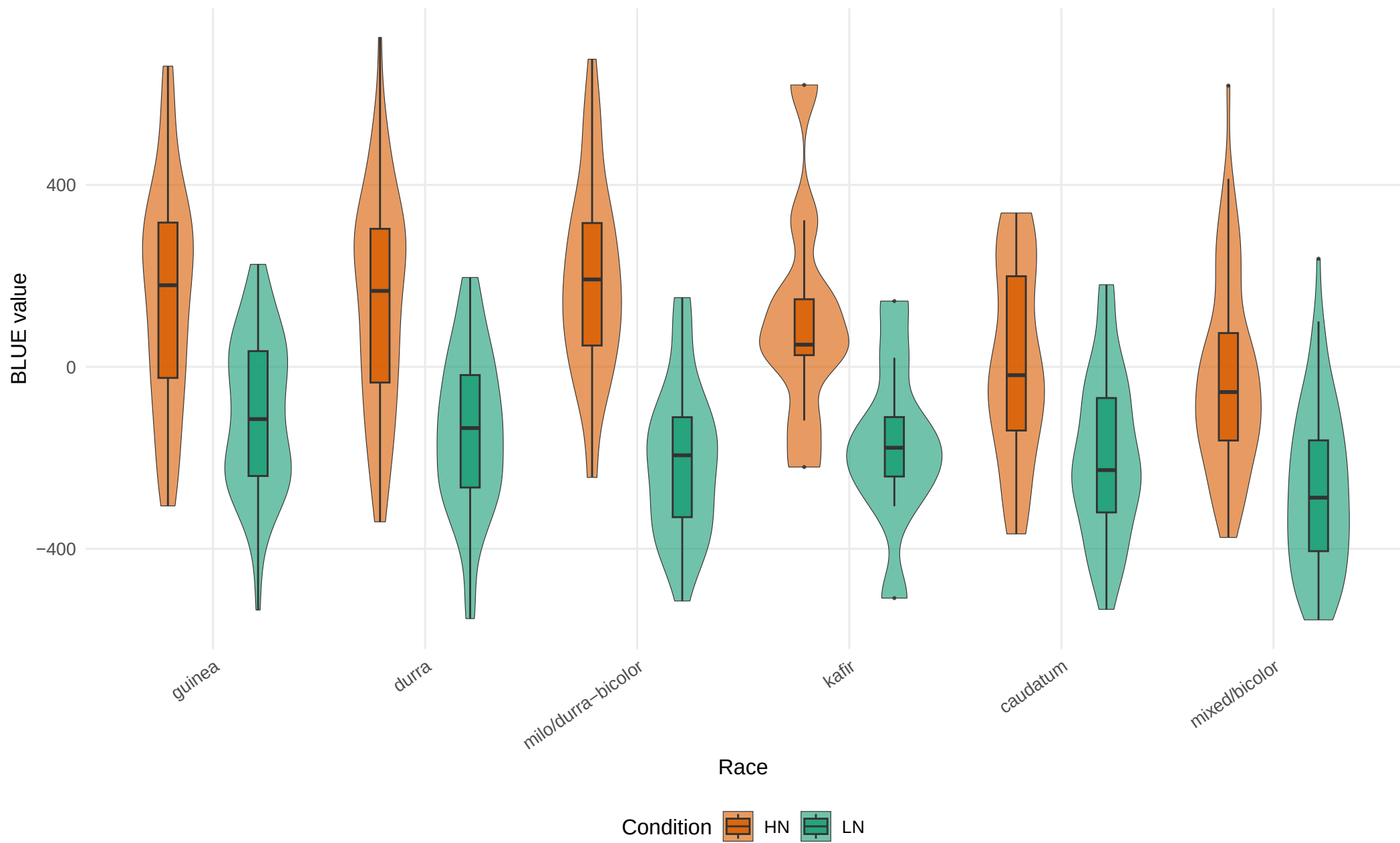
2020 | estimatedPlotYield | Violin+Box (HN vs LN)
