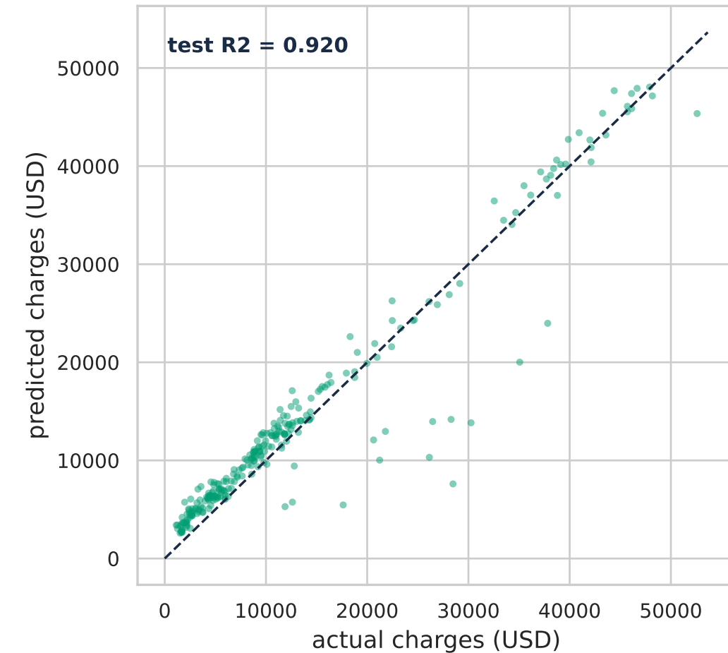
(f) Predicted vs Actual (GB)
