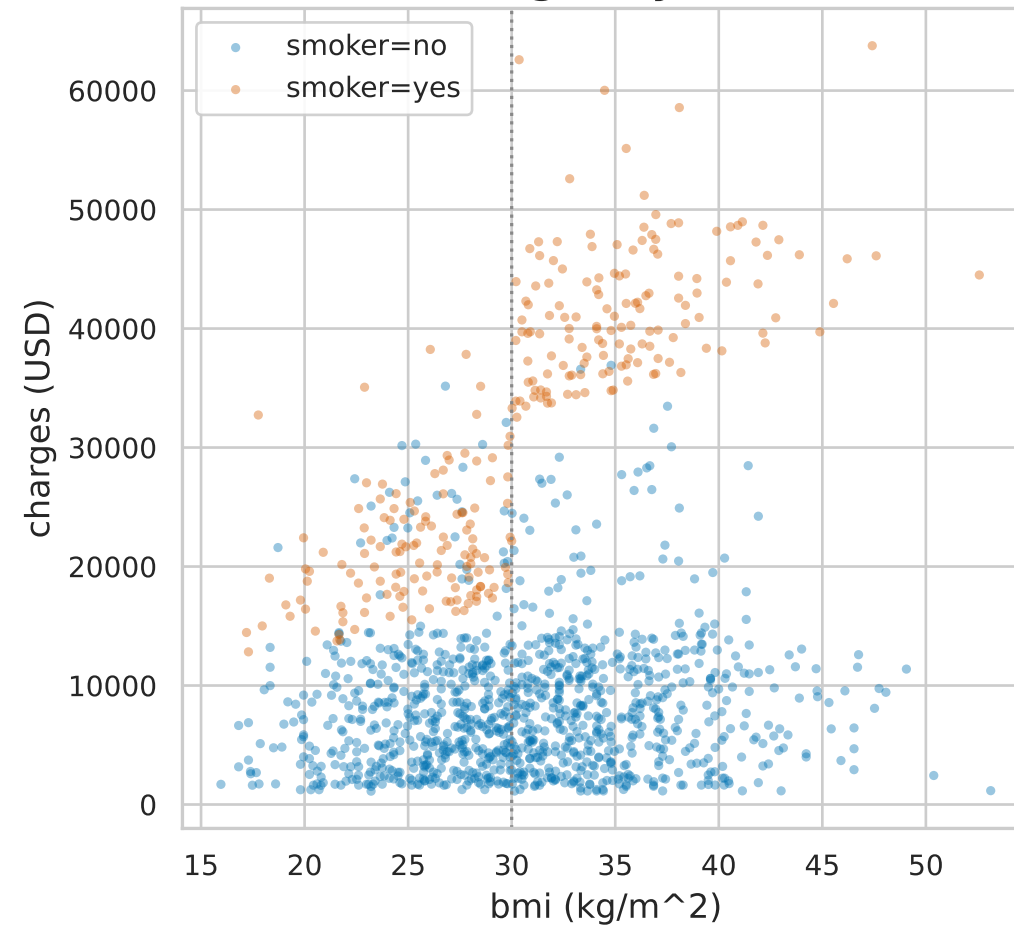
(d) BMI vs Charges by Smoker
