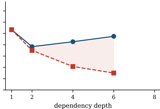
allam-2-7b
