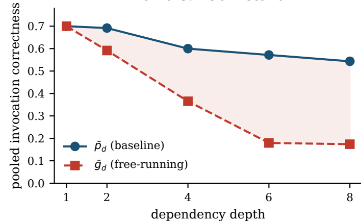
llama-3.1-8b-instant
