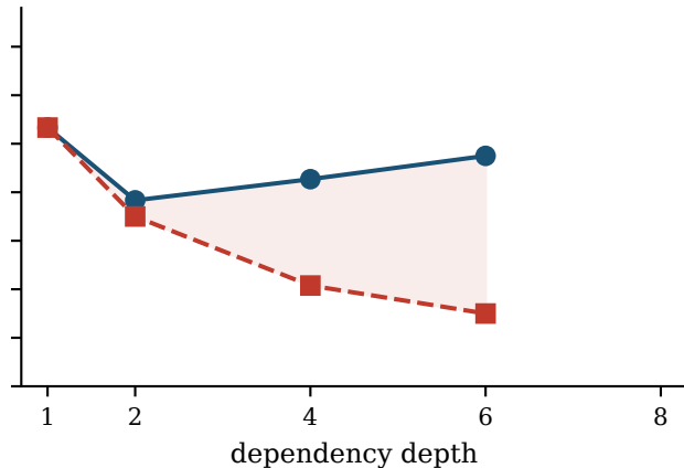
allam-2-7b
