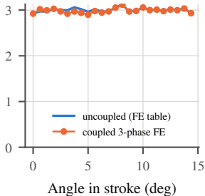
(b) Cubic TSF, 200 r/min, 3 N·m
