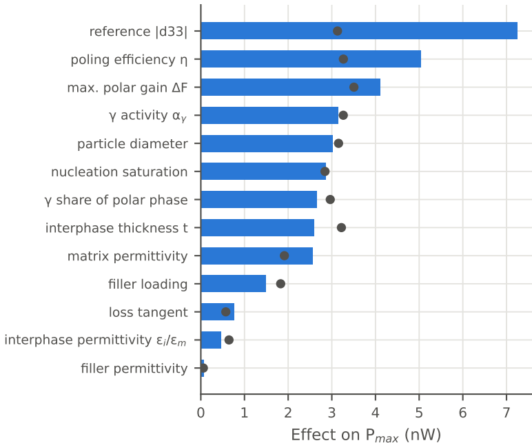
PVDF/ZnO
