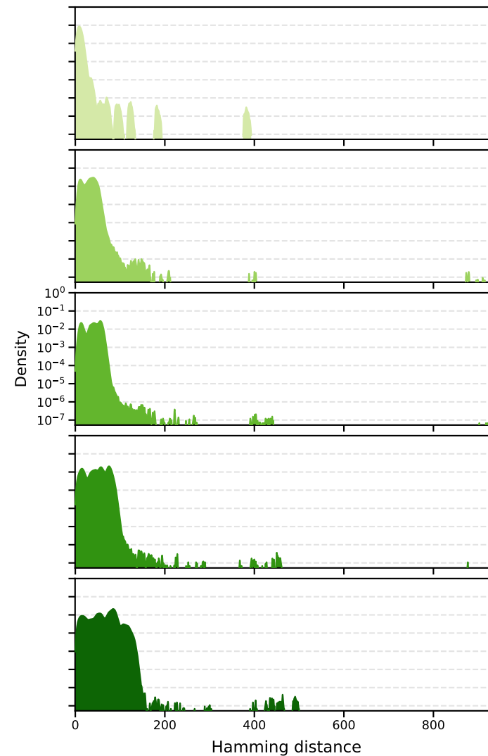
Pairwise distance
