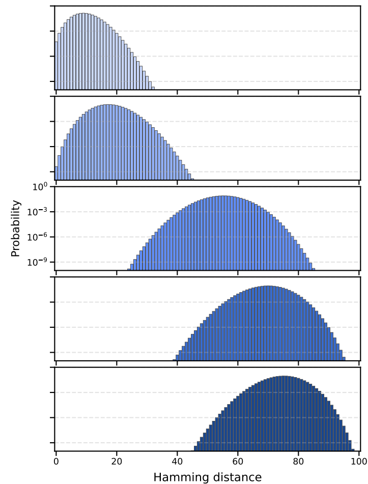
Pairwise distance
