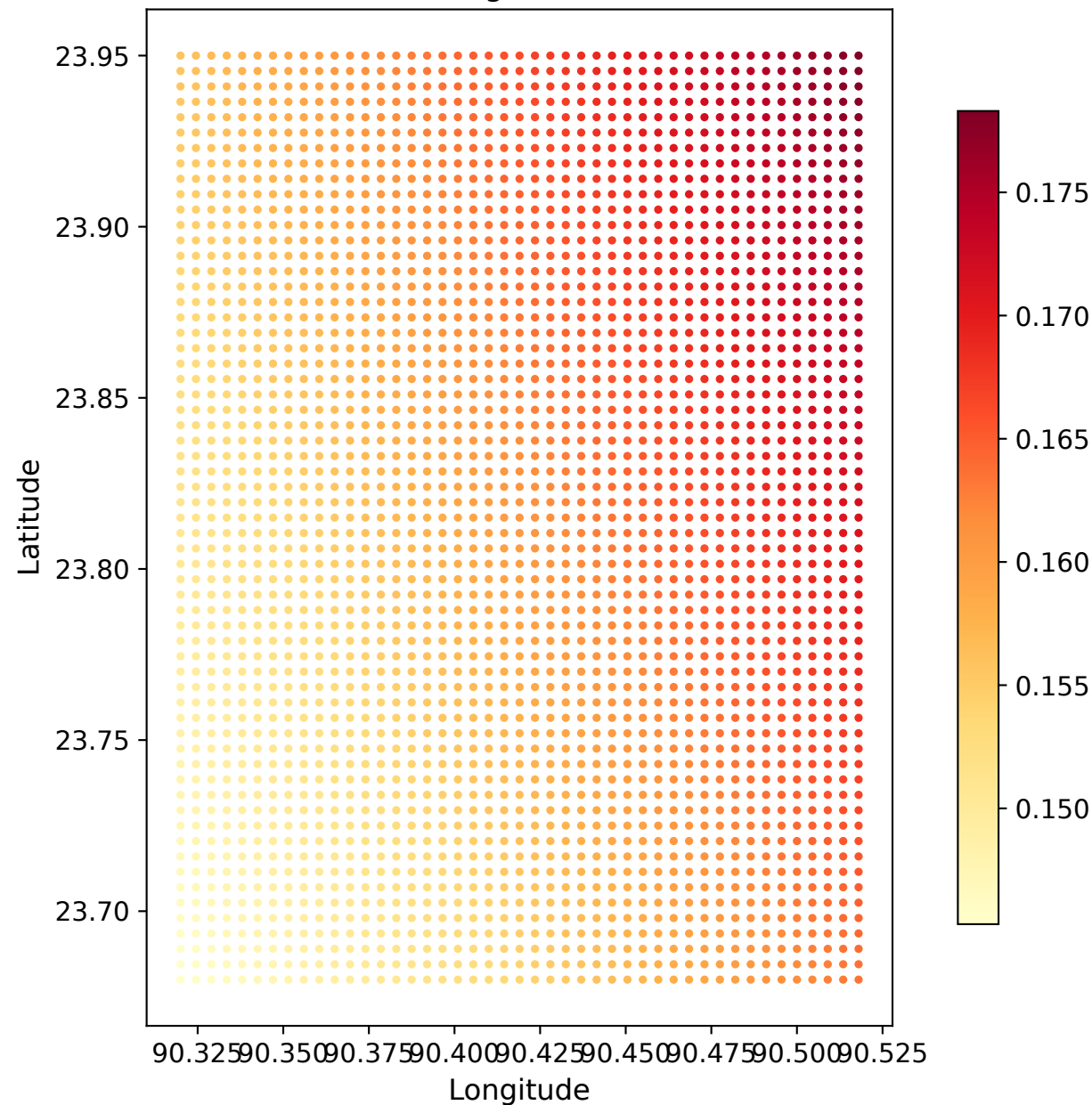
Bedrock PGA (g) — Mw 7.2 Dauki
