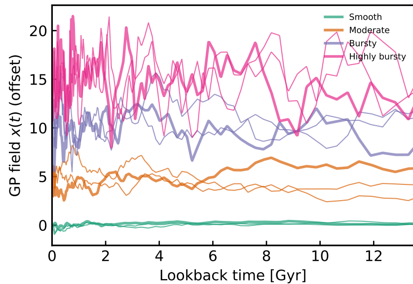
GP Realisations
