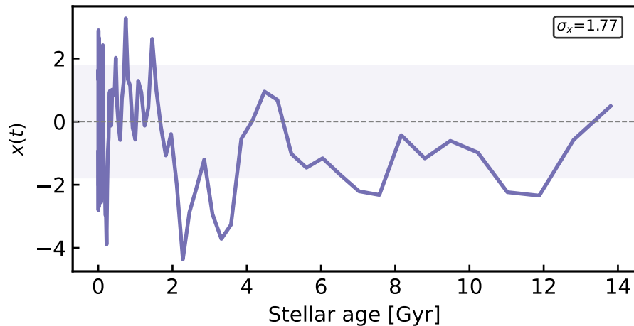
Bursty: \sigma_{\text{PS}}=2.5 , \tau_{\text{PS}}=20 Myr
