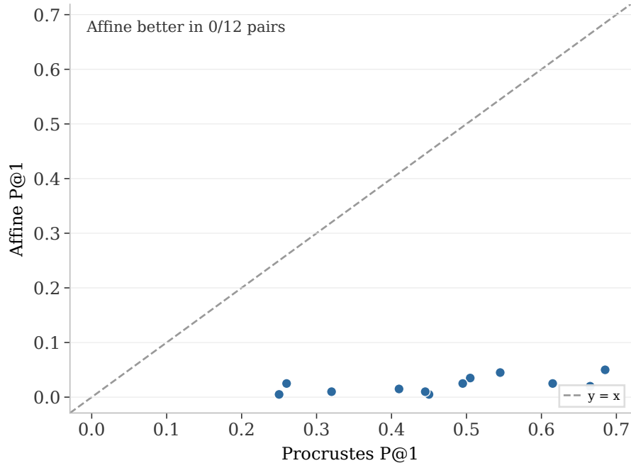
P@1
