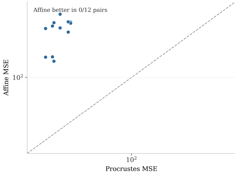
MSE
