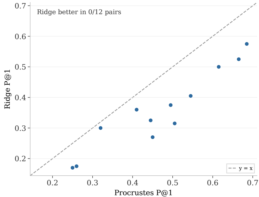
P@1
