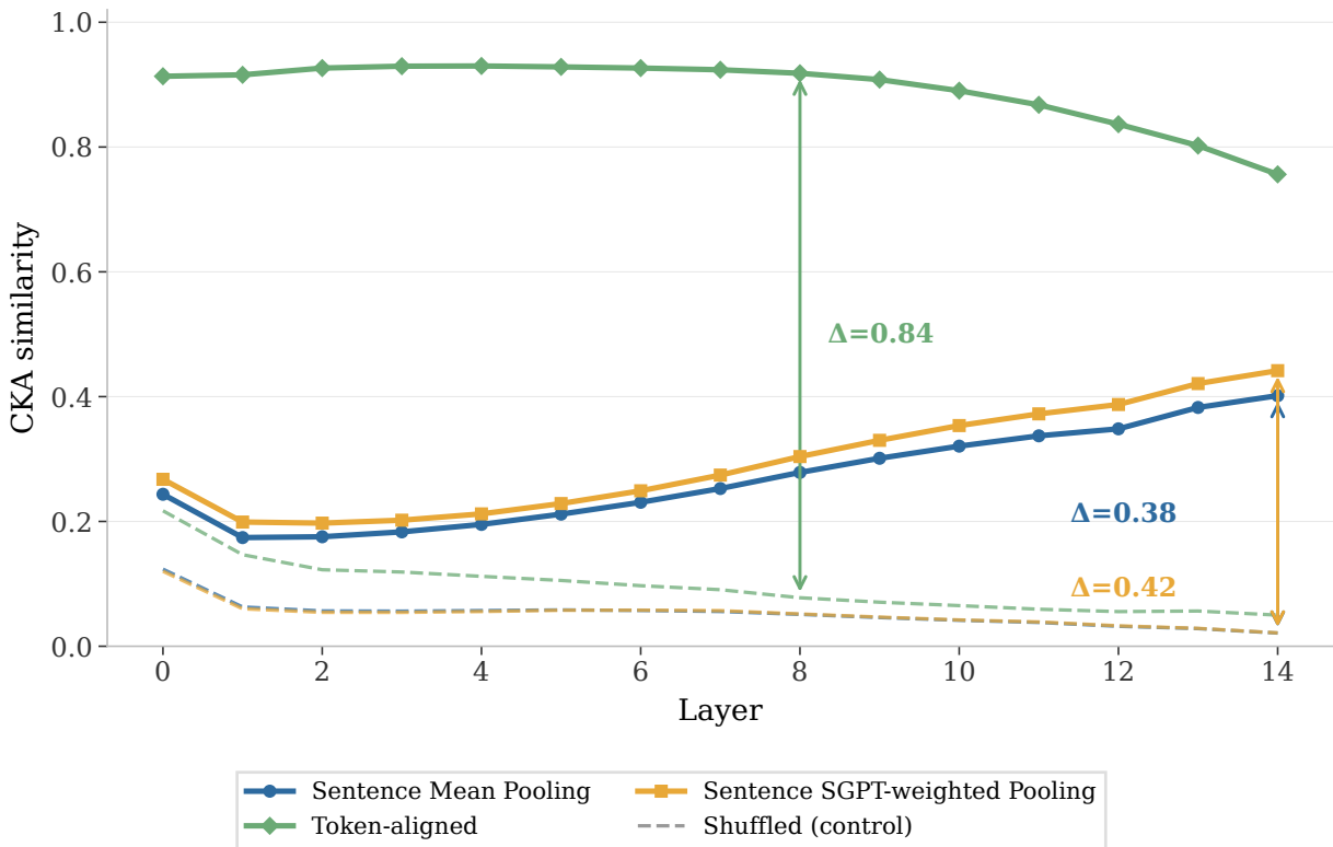
Layerwise CKA — 100M tokens
