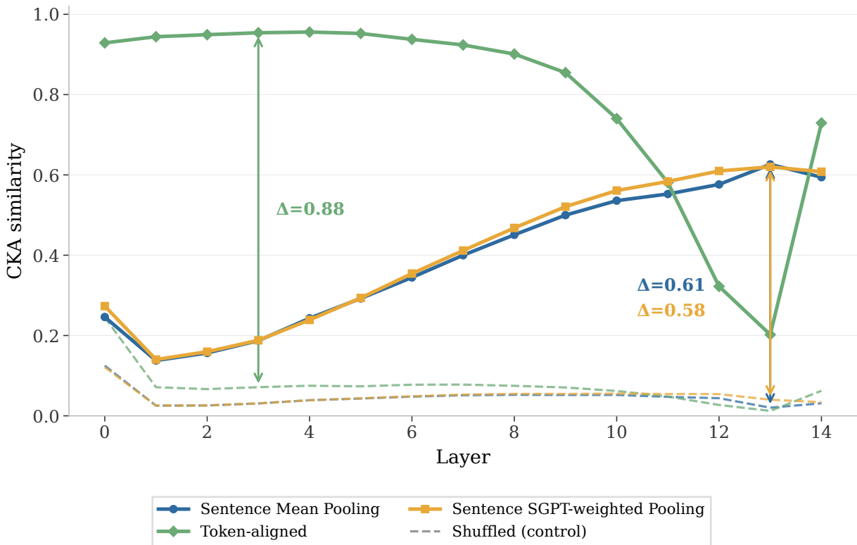
Layerwise CKA — 24B tokens
