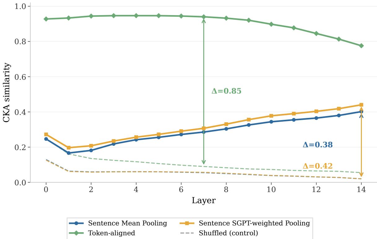
Layerwise CKA — 2B tokens
