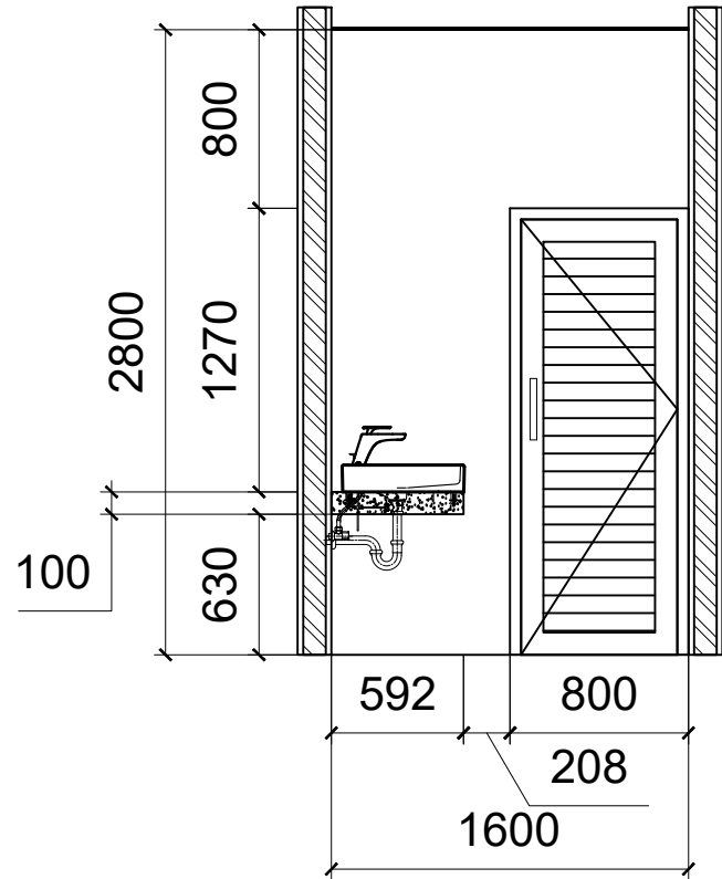
POT B-B 1:25
