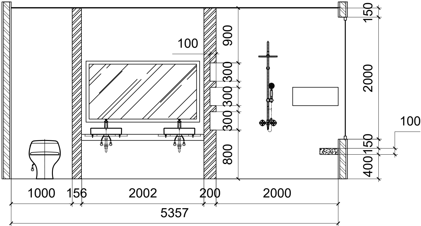
POT F-F 1:25
