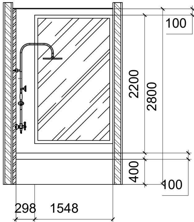
POT C-C 1:25
