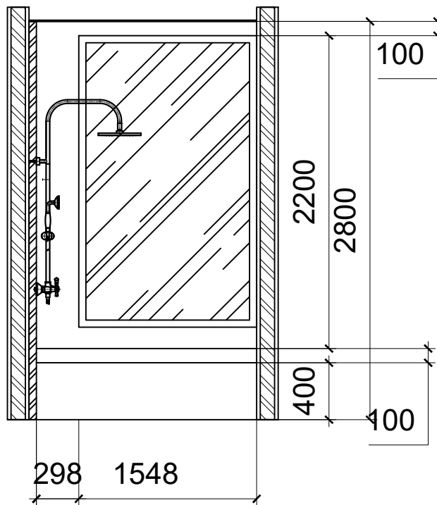
POT C-C 1:25
