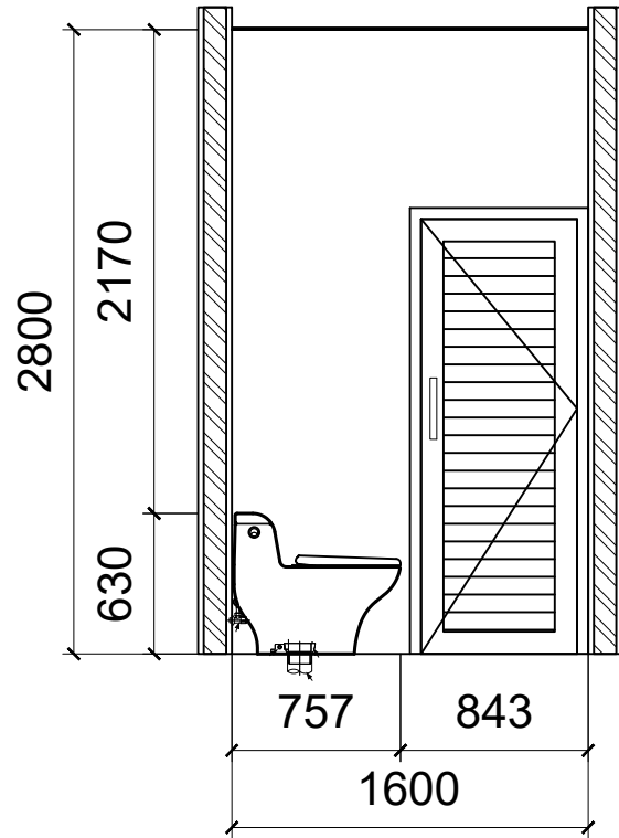
POT A-A 1:25
