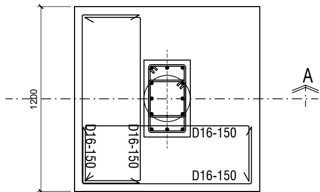
FOUNDATION DETAILS TYPE F1 SCALE 1:25
