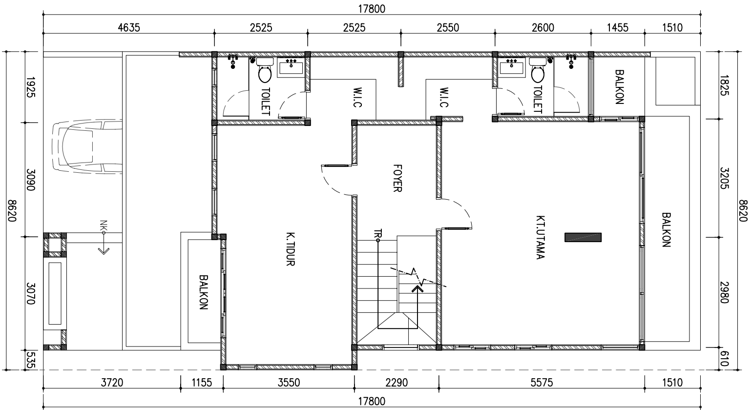
DENAH LANTAI TIGA SKALA
