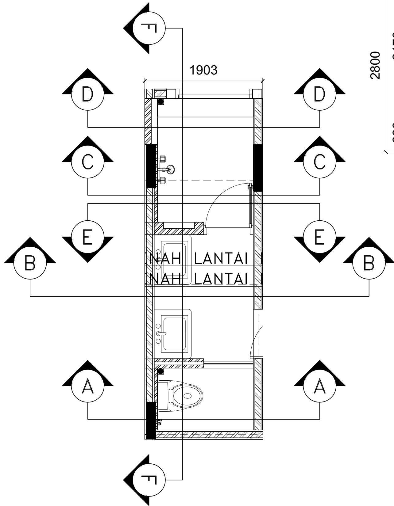
DENAH K.MANDI UTAMA 1:25
