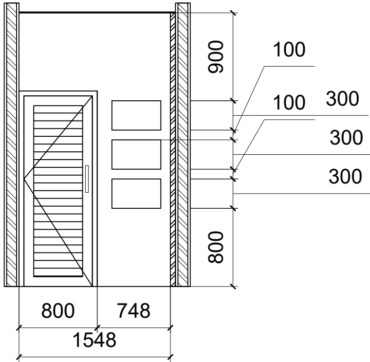
POT E-E 1:25
