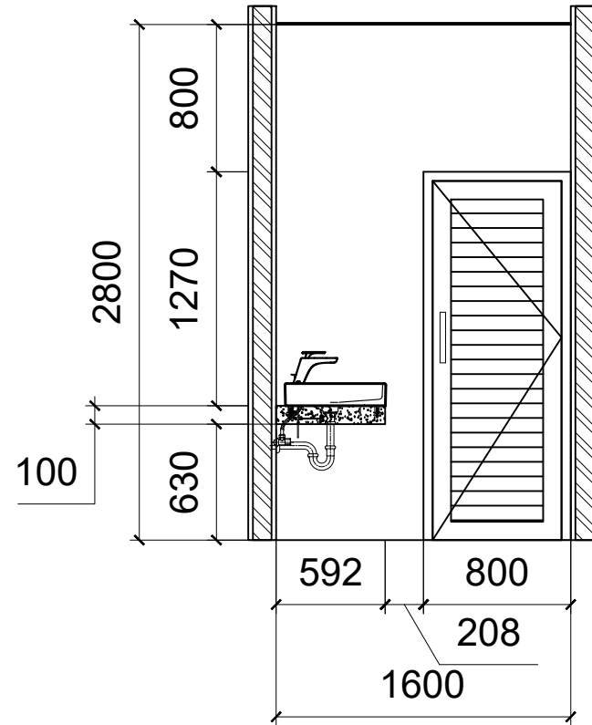
POT B-B 1:25
