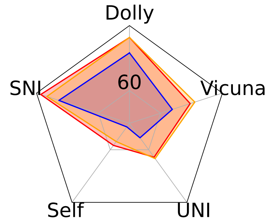
7B -> 3B
