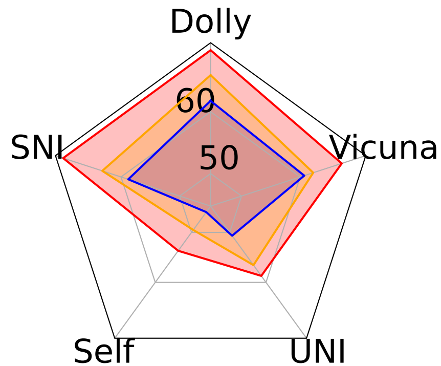
3B -> 0.5B
