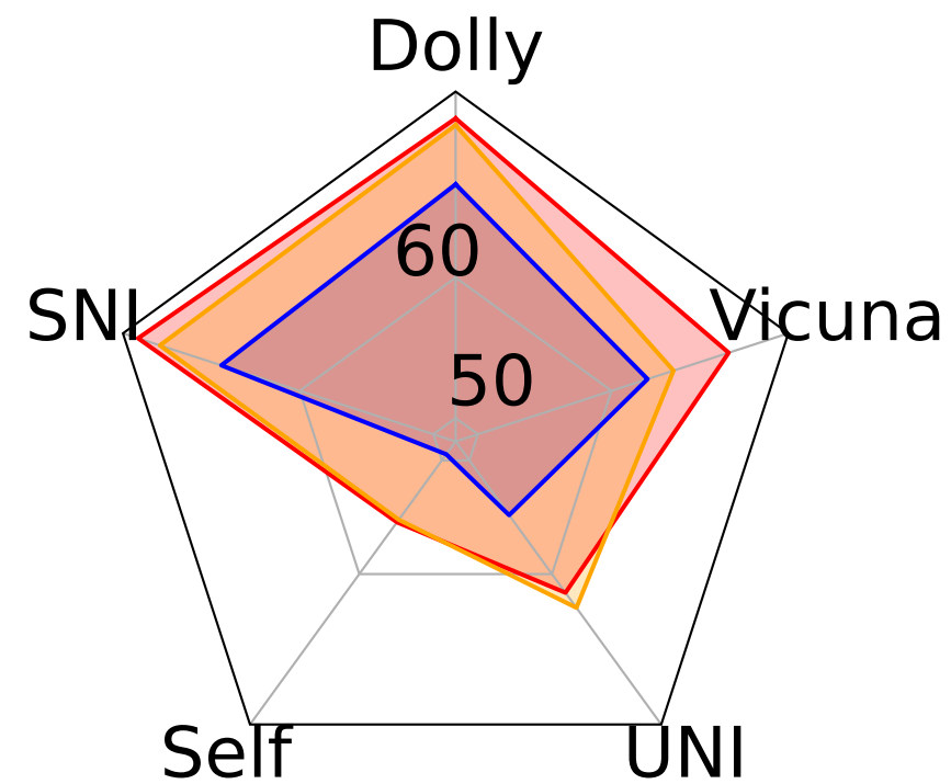
3B -> 1.5B
