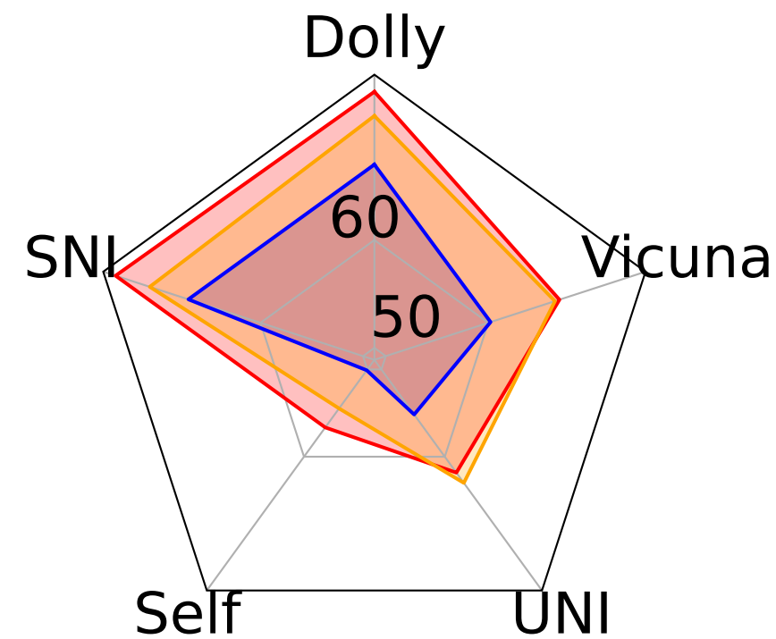
7B -> 1.5B
