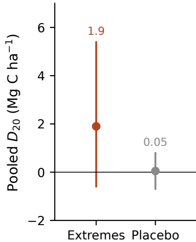
b Placebo test
