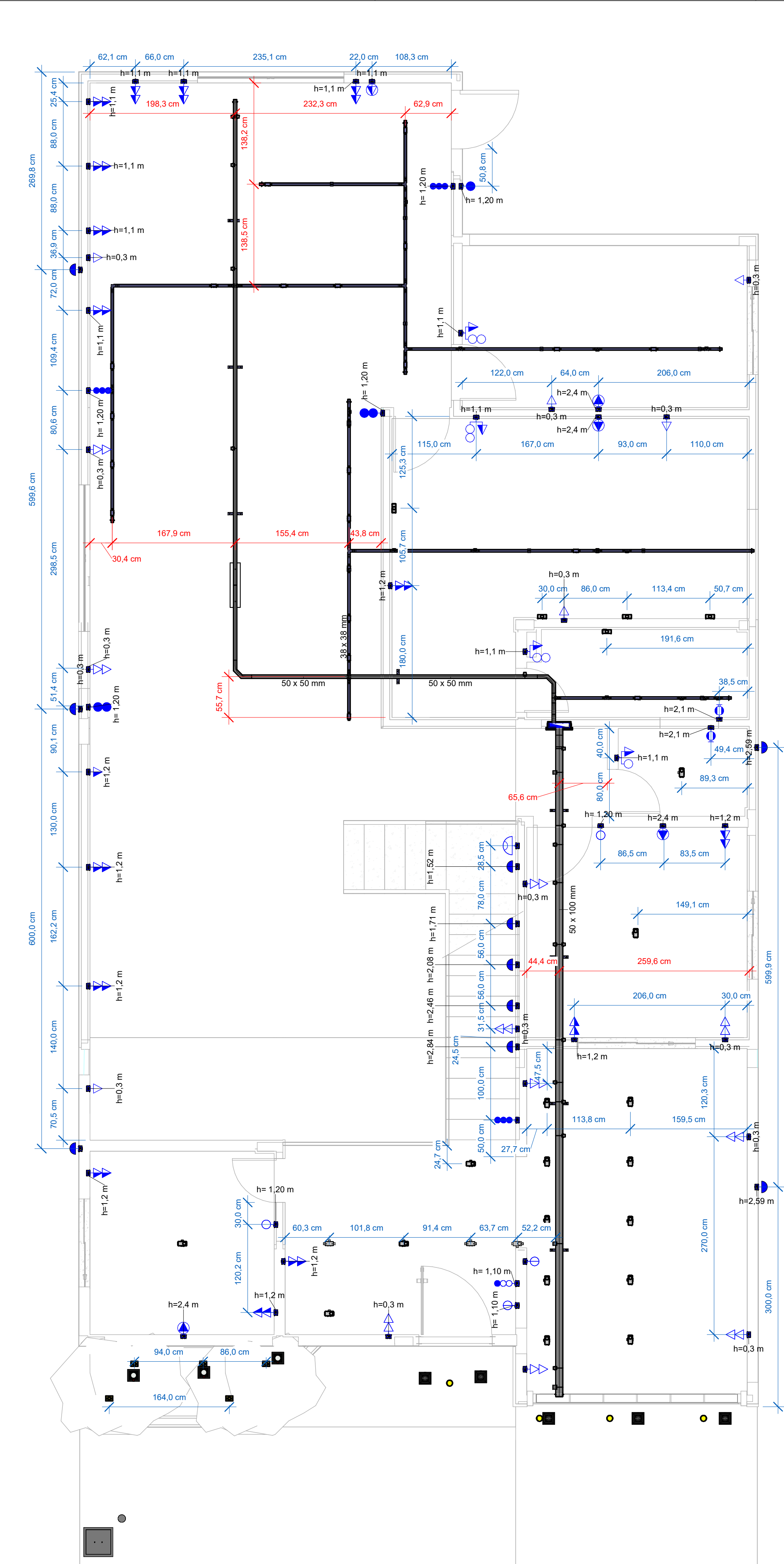
1 TÉRREO-ELT LAYOUT 1 : 40
