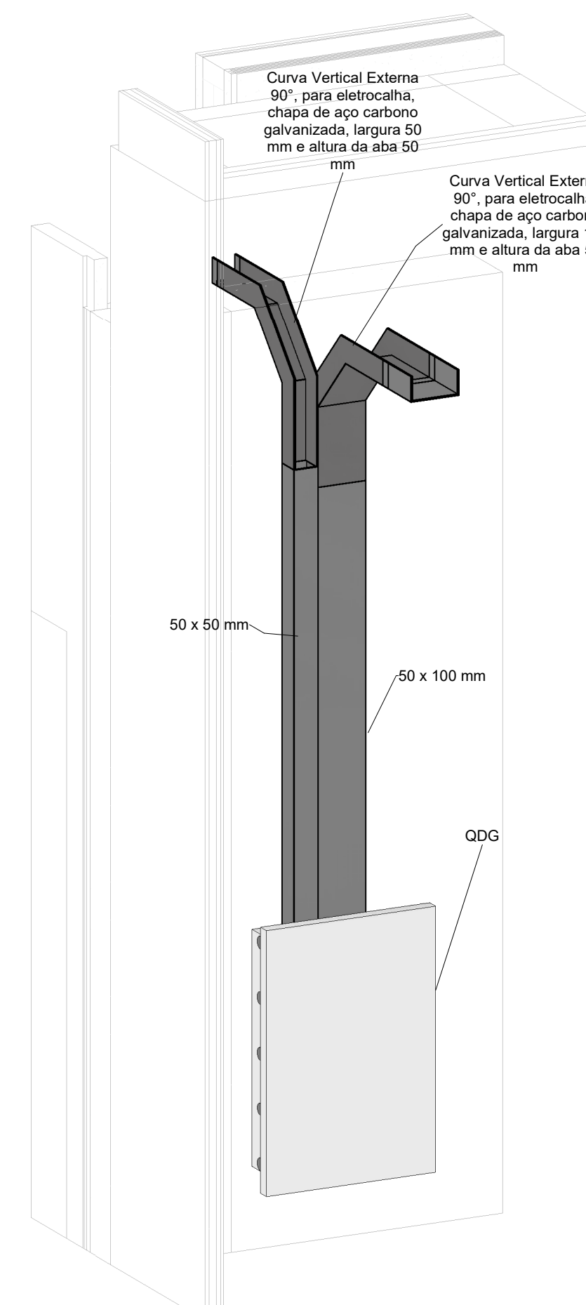
3 3D SAÍDA QUADRO
