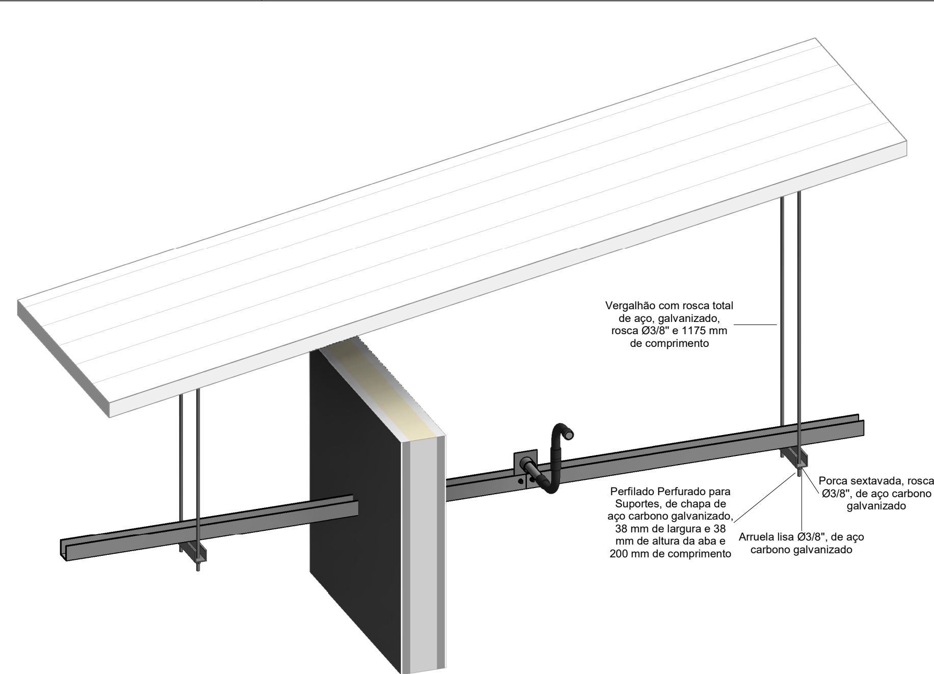
4 DETALHE SUPORTES ELETROCALHAS
