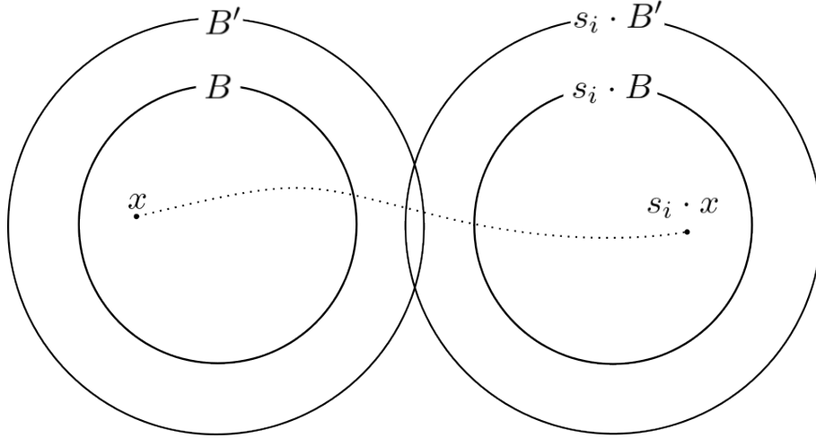
図 3: d_X(x, s_i \cdot x) の不等式
