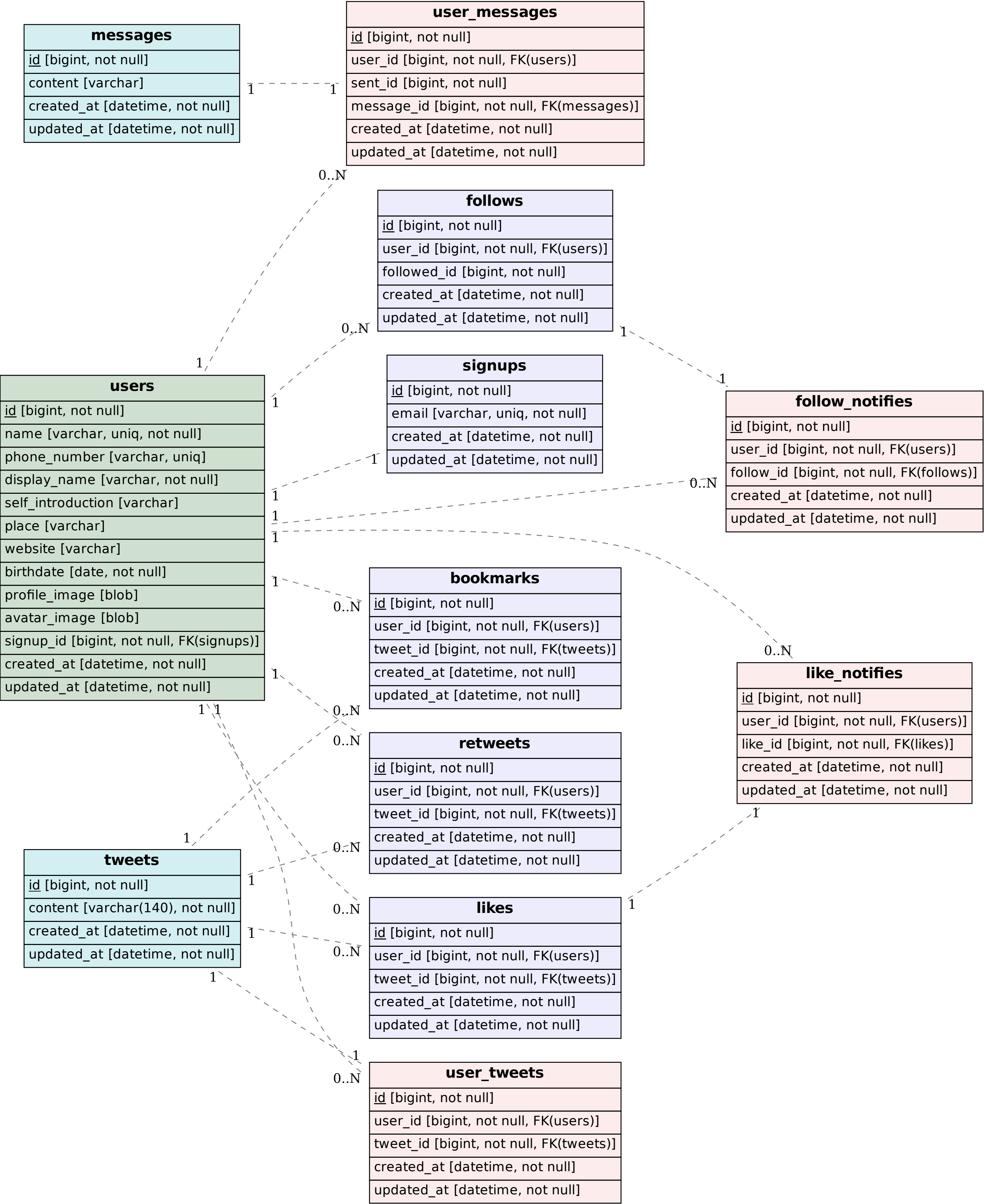
twitter ER diagram
