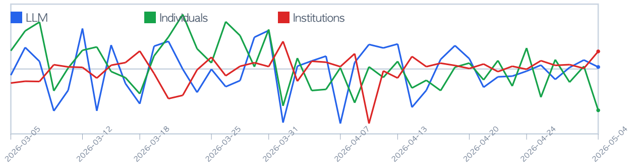
Volume MaxAbs 정규화 순거래 흐름: LLM vs 개인·기관
