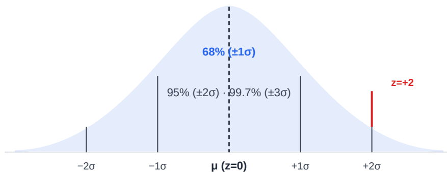
ภาพ S.2 · เส้นโค้งปกติ + กฎ 68-95-99.7 — z=+2 อยู่ขอบ 95%
