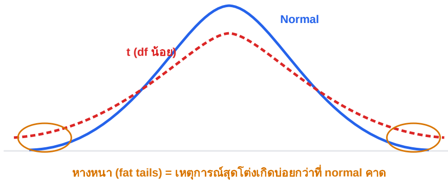
ภาพ S.3 · t-distribution หางหนากว่า normal — ตรงกับพฤติกรรมราคาคริปโต
