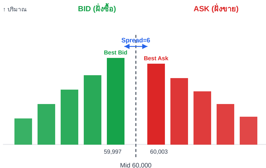
ภาพ 0.1 · กระดาน LOB (เทมเพลตแม่ของทั้งเล่ม) — เป็นภาพ schematic เพื่อสื่อแนวคิด ความสูงของแท่งไม่ใช่โปรไฟล์ depth จริง
