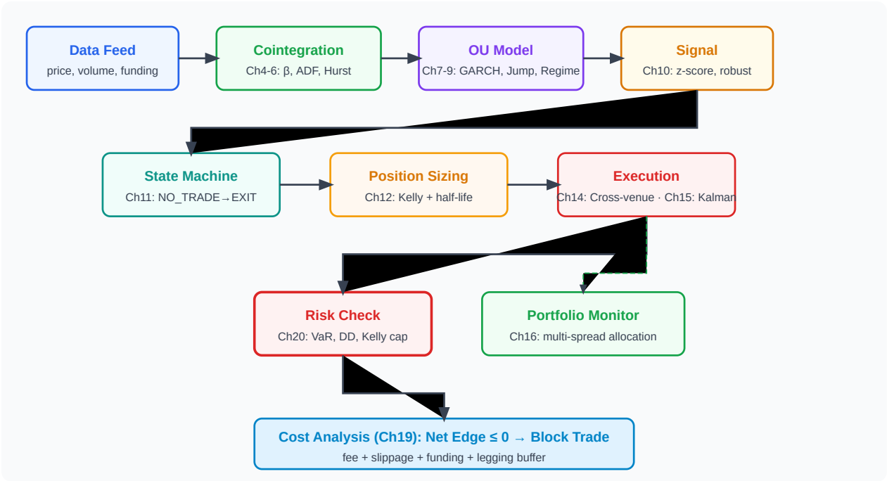
Architecture ของ Stat Arb System — ทุก module เชื่อมกันเป็น pipeline จาก data ถึง execution
