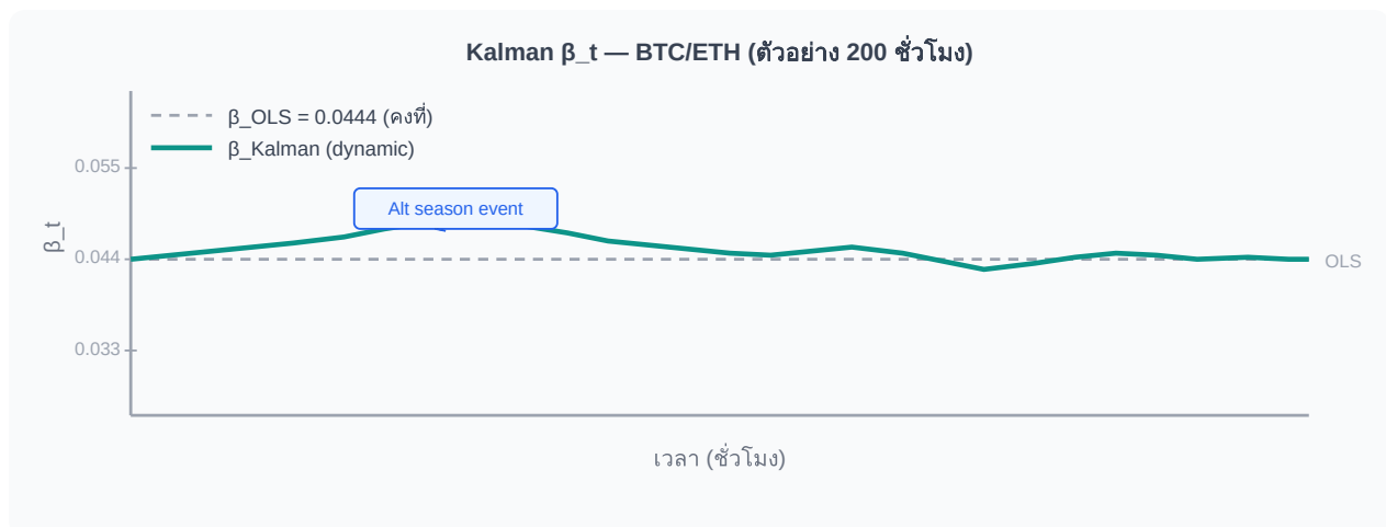
รูป 23.3 — \beta_t ของ Kalman Filter (เขียว) เพิ่มขึ้นระหว่าง altcoin season แล้วกลับสู่ระดับปกติ ขณะที่ OLS คงที่ตลอด
