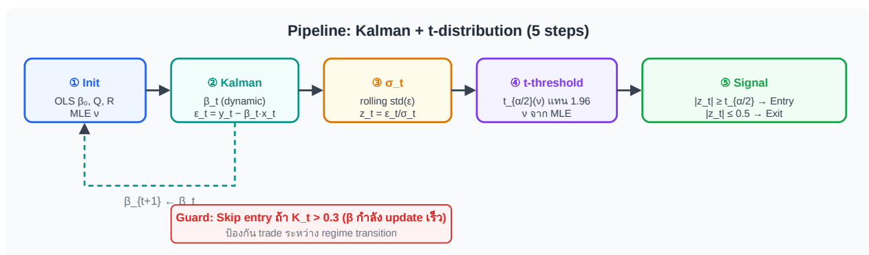
รูป 23.6 — Pipeline 5 ขั้นตอน: Kalman ให้ \beta_t แม่นยำ → t-distribution กำหนด threshold ที่เหมาะสม
