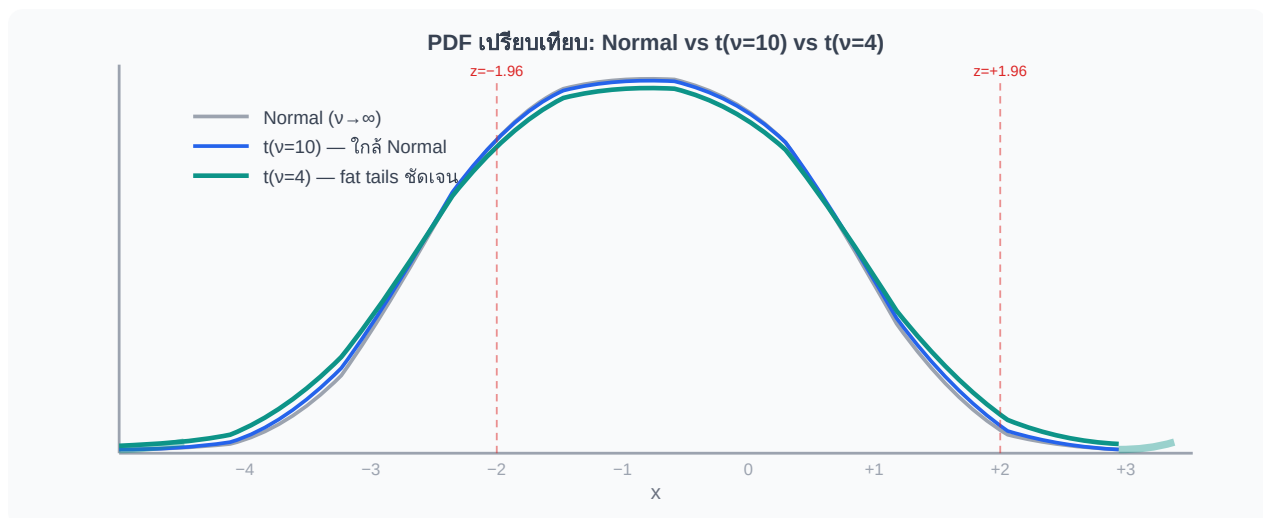
รูป 23.5 — t( \nu=4 ) มีหางหนักกว่า Normal ชัดเจน — area นอก \pm 1.96 ใหญ่กว่า 2\times สำหรับ crypto \nu \approx 3-6
