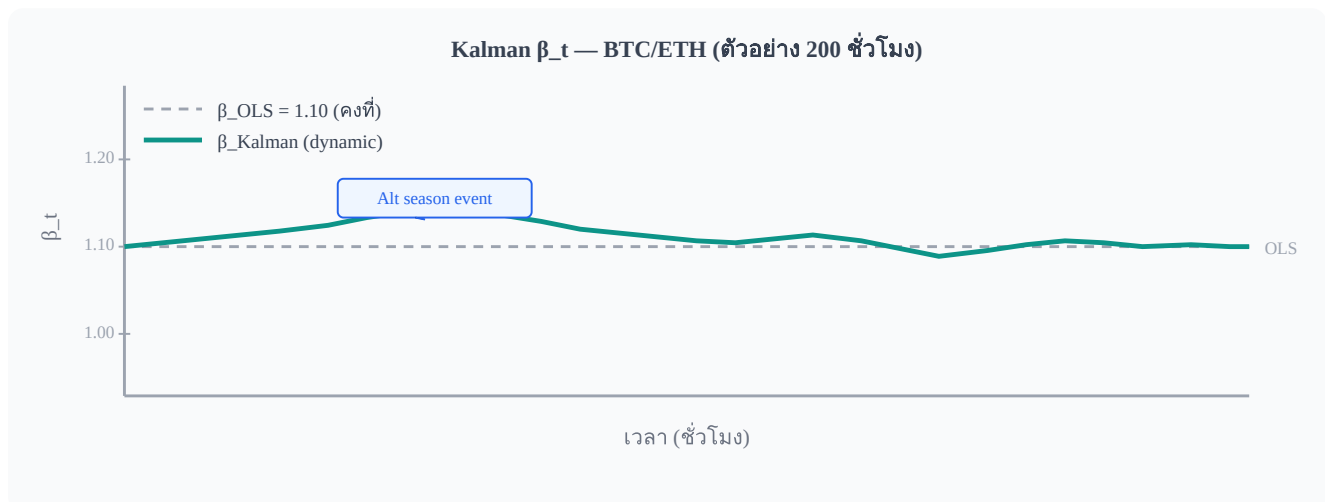
รูป 23.3 — \beta_t ของ Kalman Filter (เขียว) เคลื่อนขึ้นระหว่าง altcoin season แล้วกลับสู่ระดับปกติ ขณะที่ OLS คงที่ตลอด (log-return scale: \beta \approx 1.0\text{--}1.2 )
