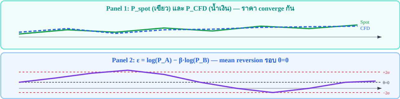
Panel บน: P_{spot} และ P_{CFD} เคลื่อนที่ใกล้กัน | Panel ล่าง: \epsilon oscillates รอบ \theta=0 ภายใน \pm 2\sigma band
