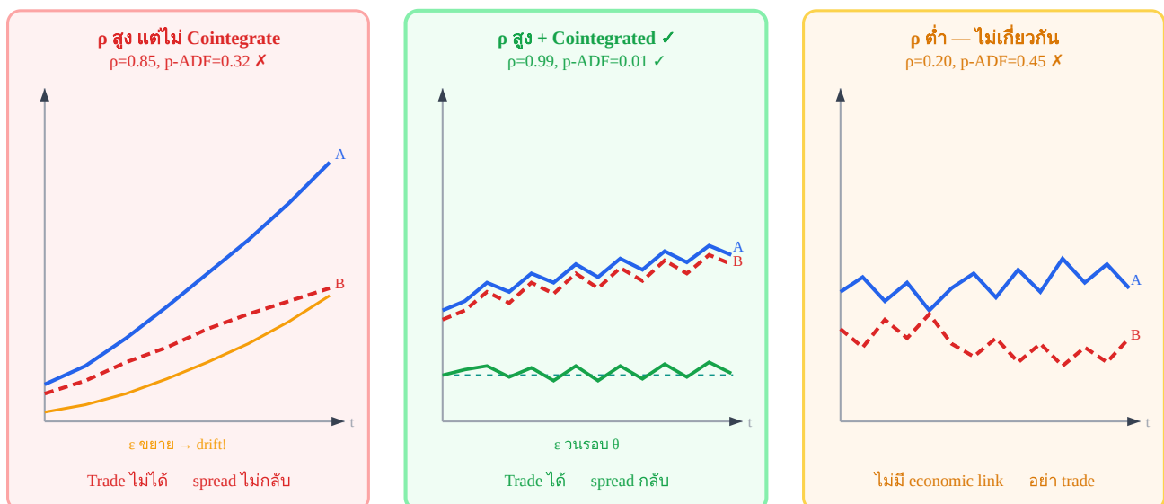
3 สถานการณ์ — Correlation และ Cointegration
