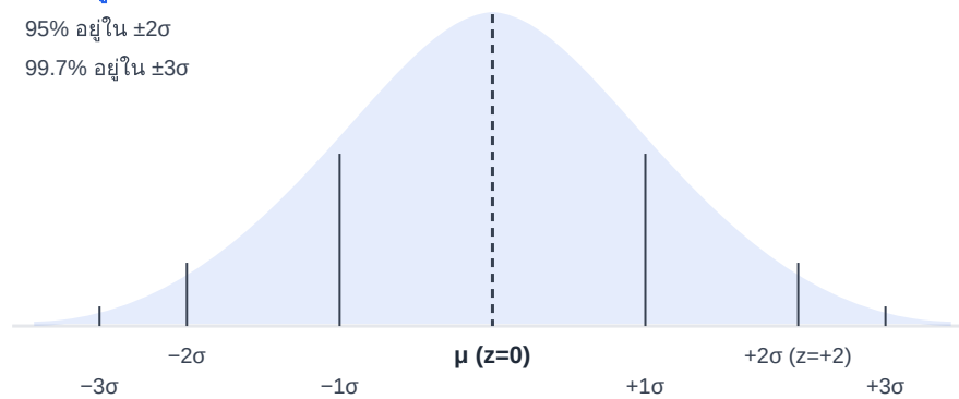
ภาพ S.2 · เส้นโค้งปกติ + กฎ 68-95-99.7 — z=+2 ตรงกับขอบ \pm 2\sigma (ครอบคลุม 95%)
