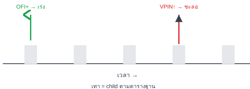
ภาพ EX3.2 · สัญญาณกระดานไม่ล้มนตาราง — แคขยับ child ถัดไปให้เร็วขึ้น (flow หนุน) หรือช้าลง (toxic)
