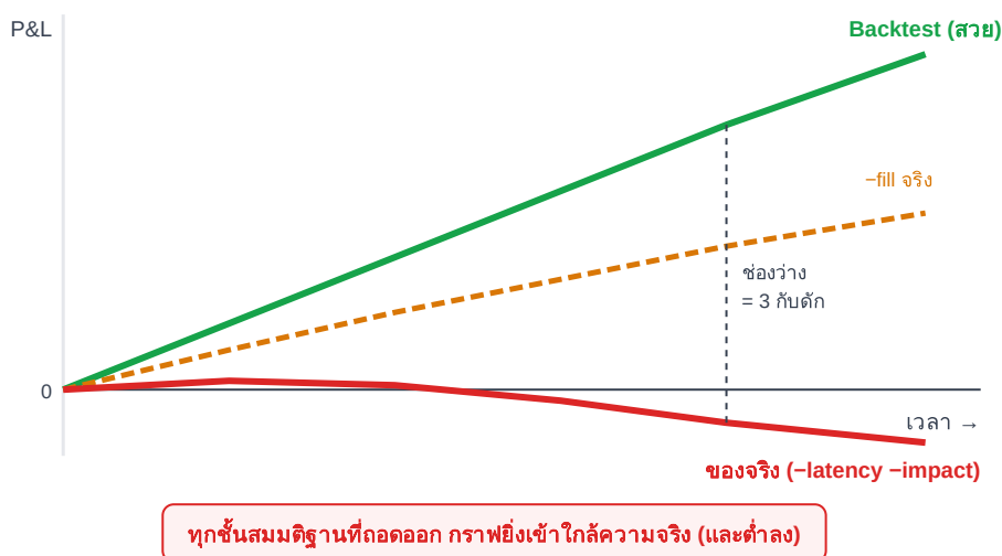
ภาพ 11.2 · backtest สวอย vs ความจริง — fill assumption + latency + market impact กินกำไรหมด
