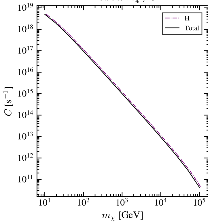
AGSS09: c_4^0 \neq 0
