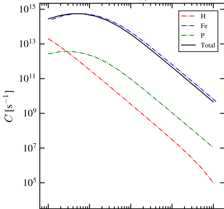
AGSS09: c_8^0 \neq 0
