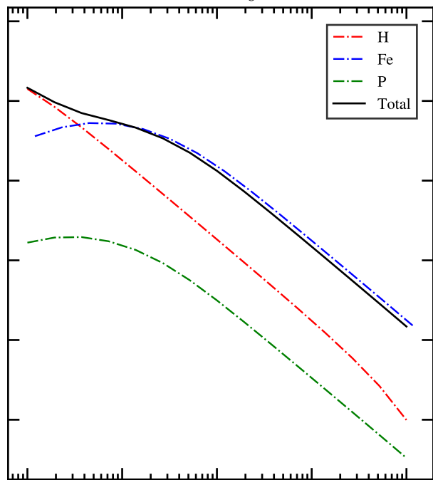
AGSS09: c_8^1 \neq 0
