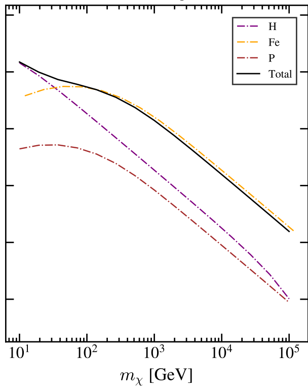
AGSS09: c_8^1 \neq 0
