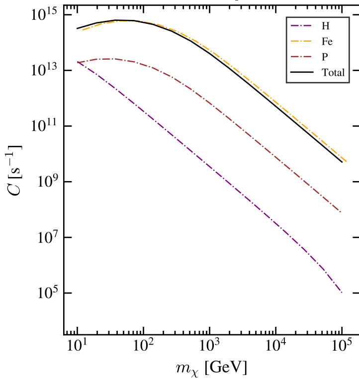
AGSS09: c_8^0 \neq 0
