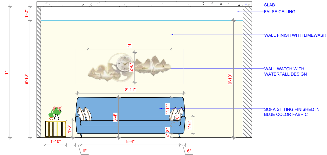
ELEVATION B
