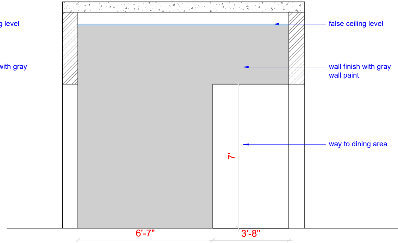
ELEVATION WALL (D)
