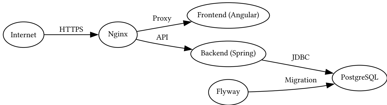
Fig. 11. – Architecture physique et logique de l'infrastructure PIAWEB
